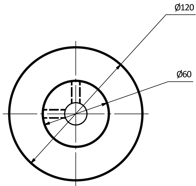
Driving wheel ( 1 : 2 ) Matière : aluminium
