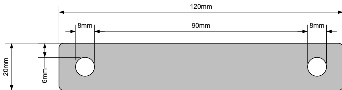
Acier épaisseur 3 mm – 4x
