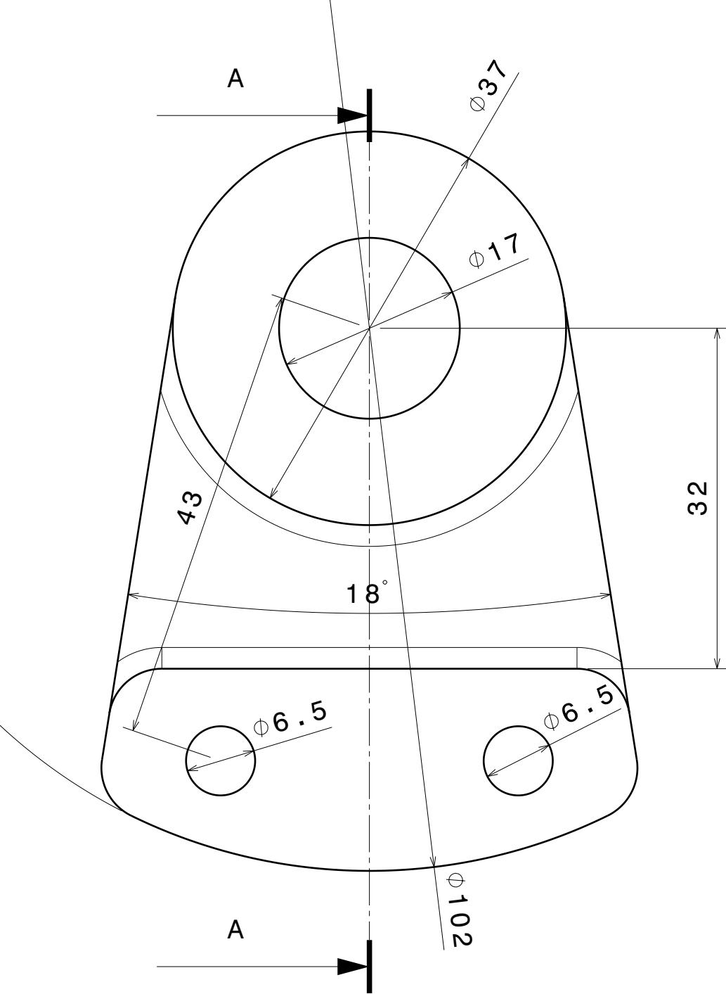
Vue de face Echelle : 2:1
