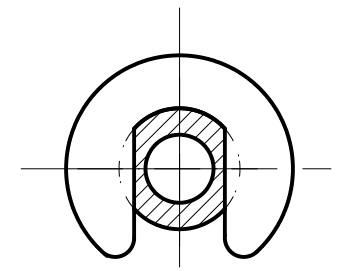
Cale montéel sur canon Soudure côté partie longue du canon
