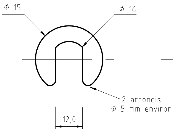
Cale - épaisseur 2 mm
