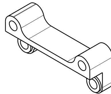
Vue isométrique Echelle : 1:2
