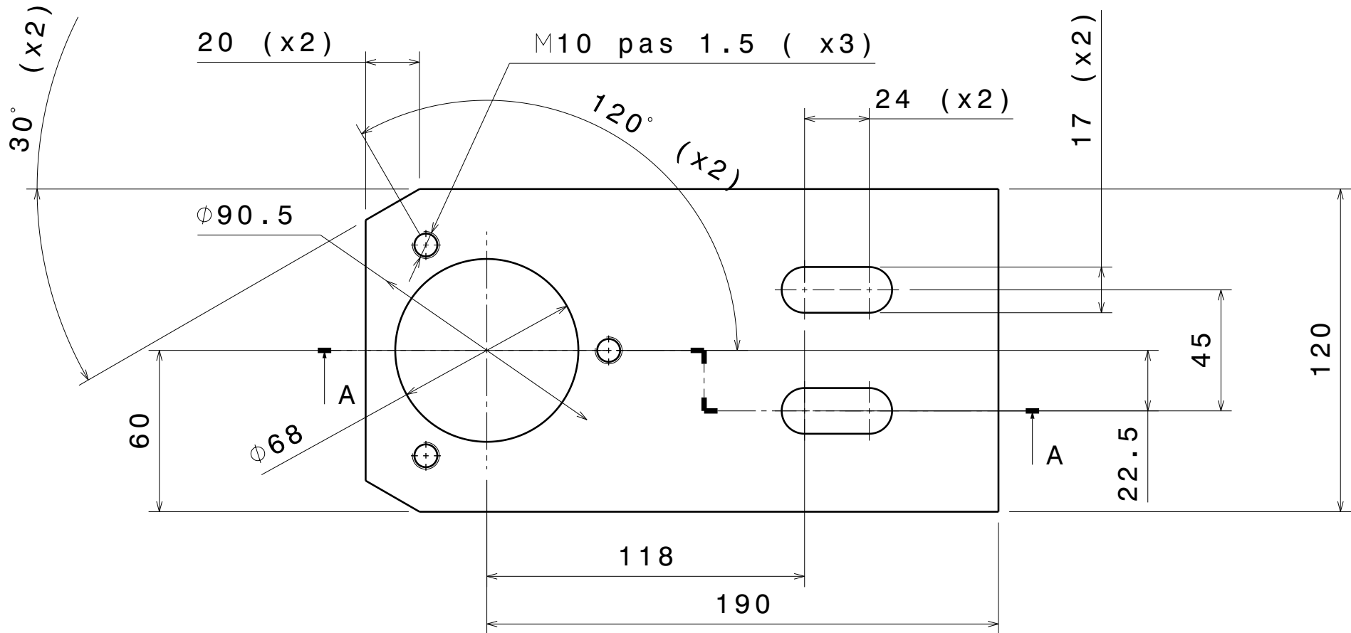
Vue de face Echelle : 1:2
