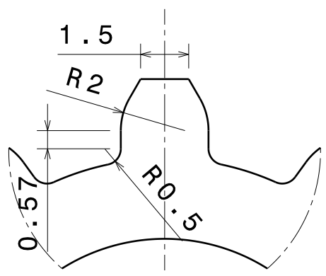
Détail A Echelle : 6:1
