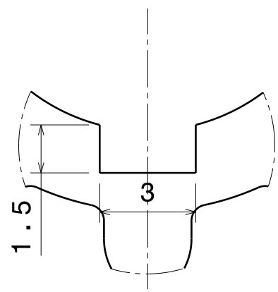
Détail B Echelle : 6:1
