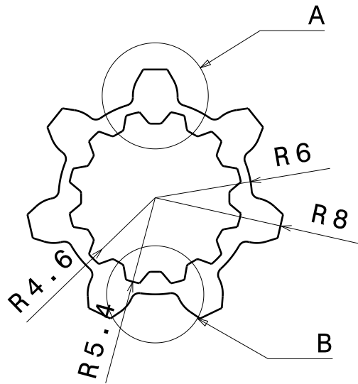
Vue de face Echelle : 3:1
