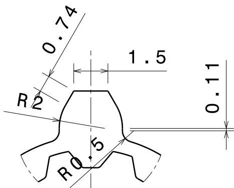
Détail A Echelle : 6:1
