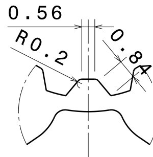
Détail B Echelle : 6:1
