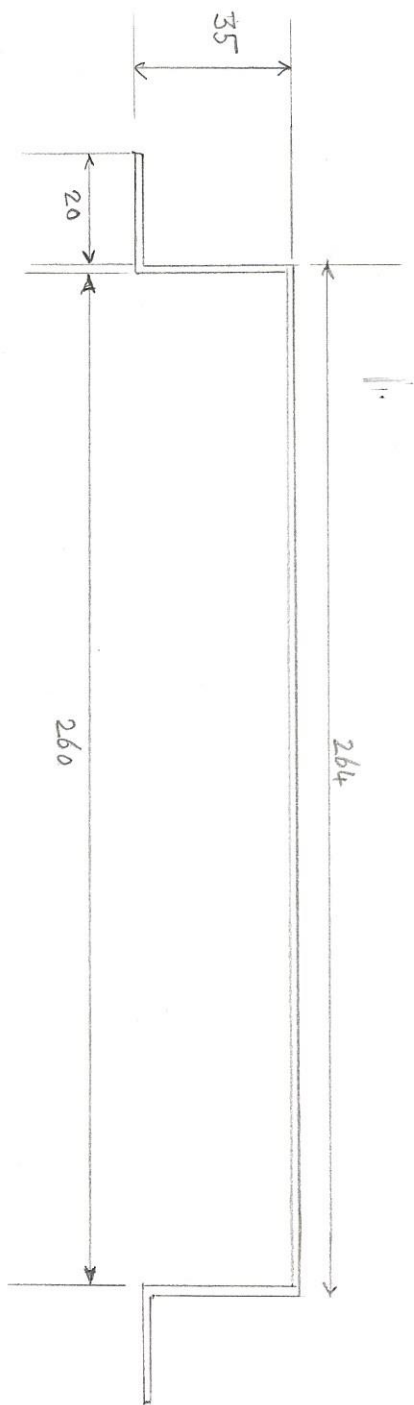
PLAQUE 1 ÉLEVATION
