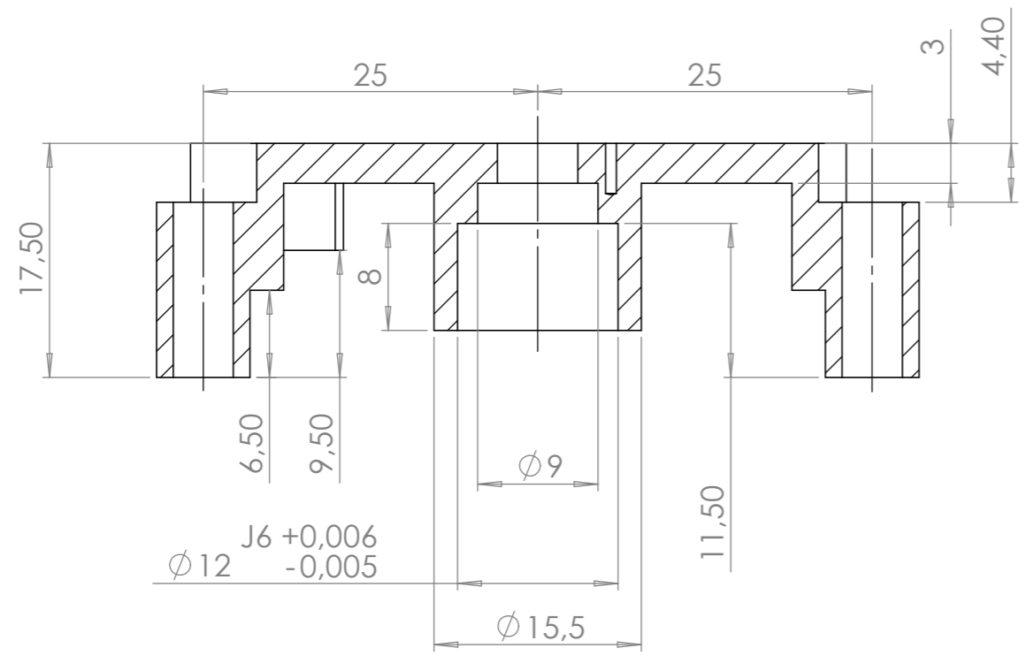
COUPE A-A
