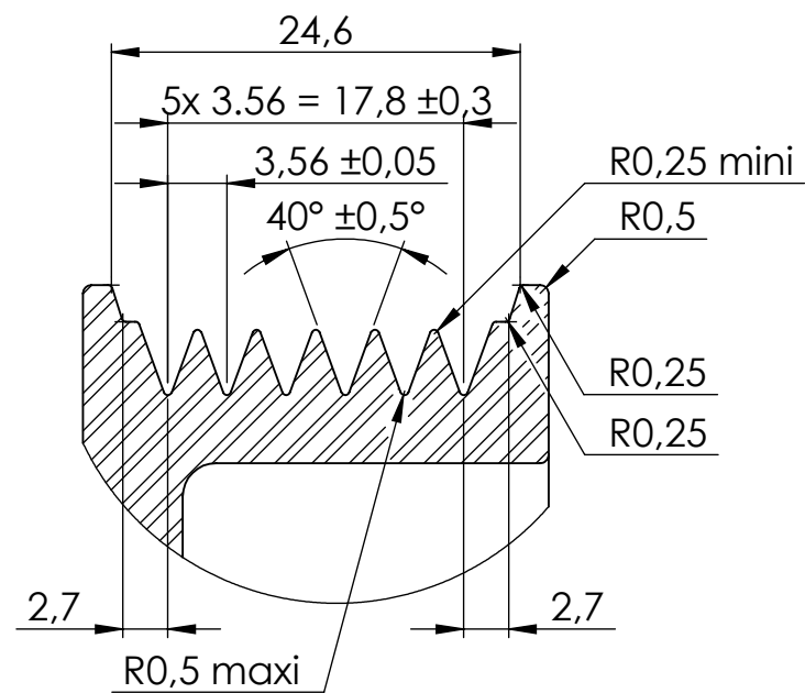
DÉTAIL B ECHELLE 2 : 1
