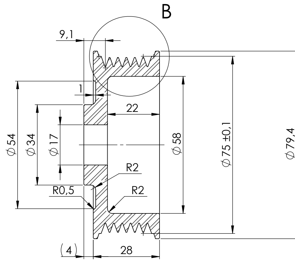
COUPE A-A
