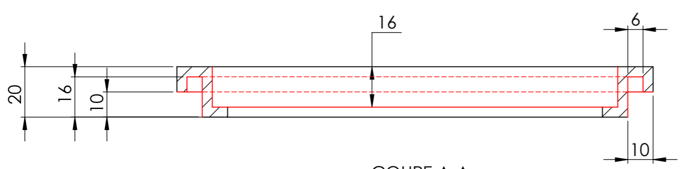
COUPE A-A ECHELLE 1 : 1.5
