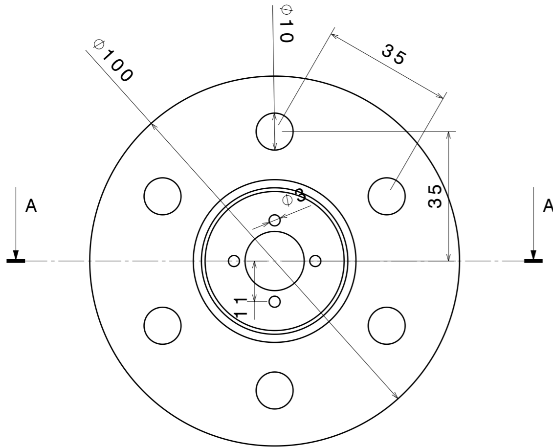
Vue de face Echelle : 1:1
