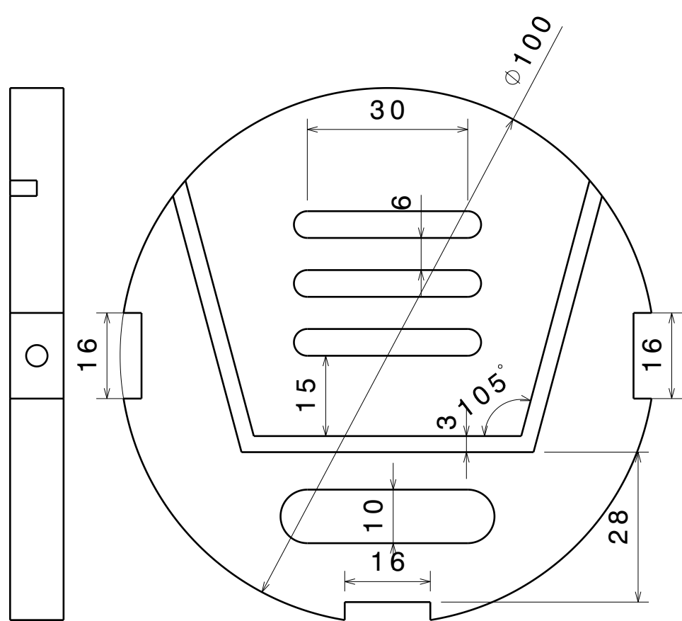
Vue de droite Echelle : 1:1
