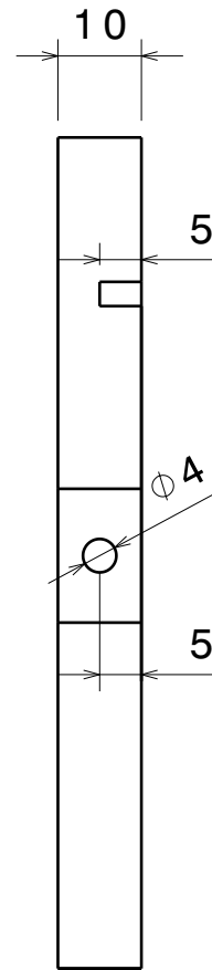
Vue de gauche Echelle : 1:1
