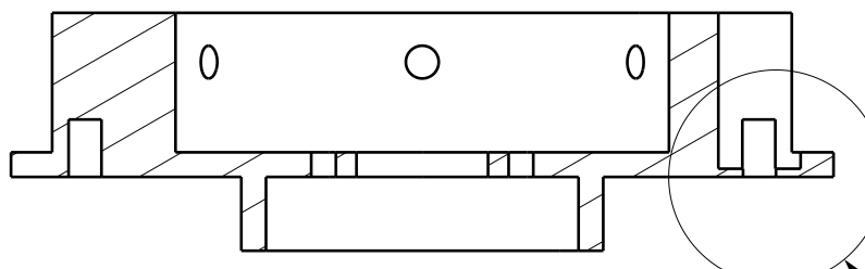
Coupe A-A Echelle : 1:1
