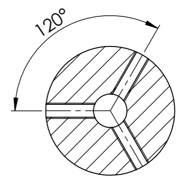
COUPE B-B ECHELLE 2 : 3
