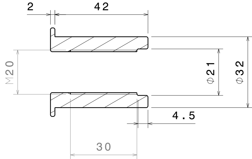
Entretoise Matiere : 7075 Qté : 1
