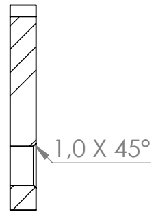
COUPE A-A
