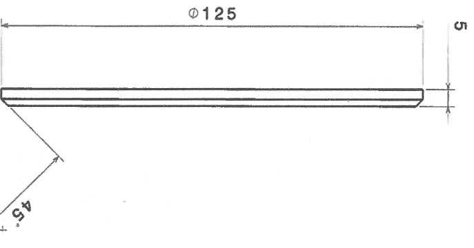
Vue de gauche Echelle : 1:1
